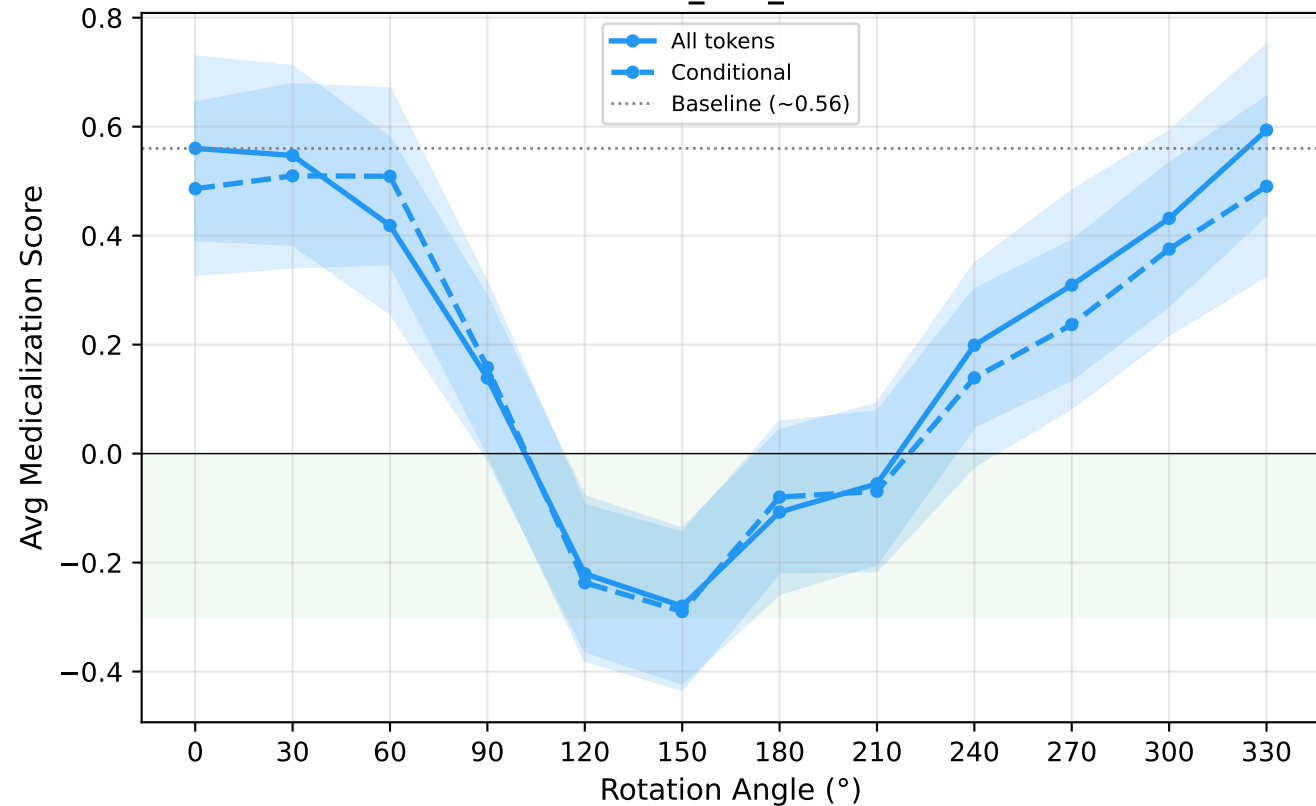
max_sim_L23
