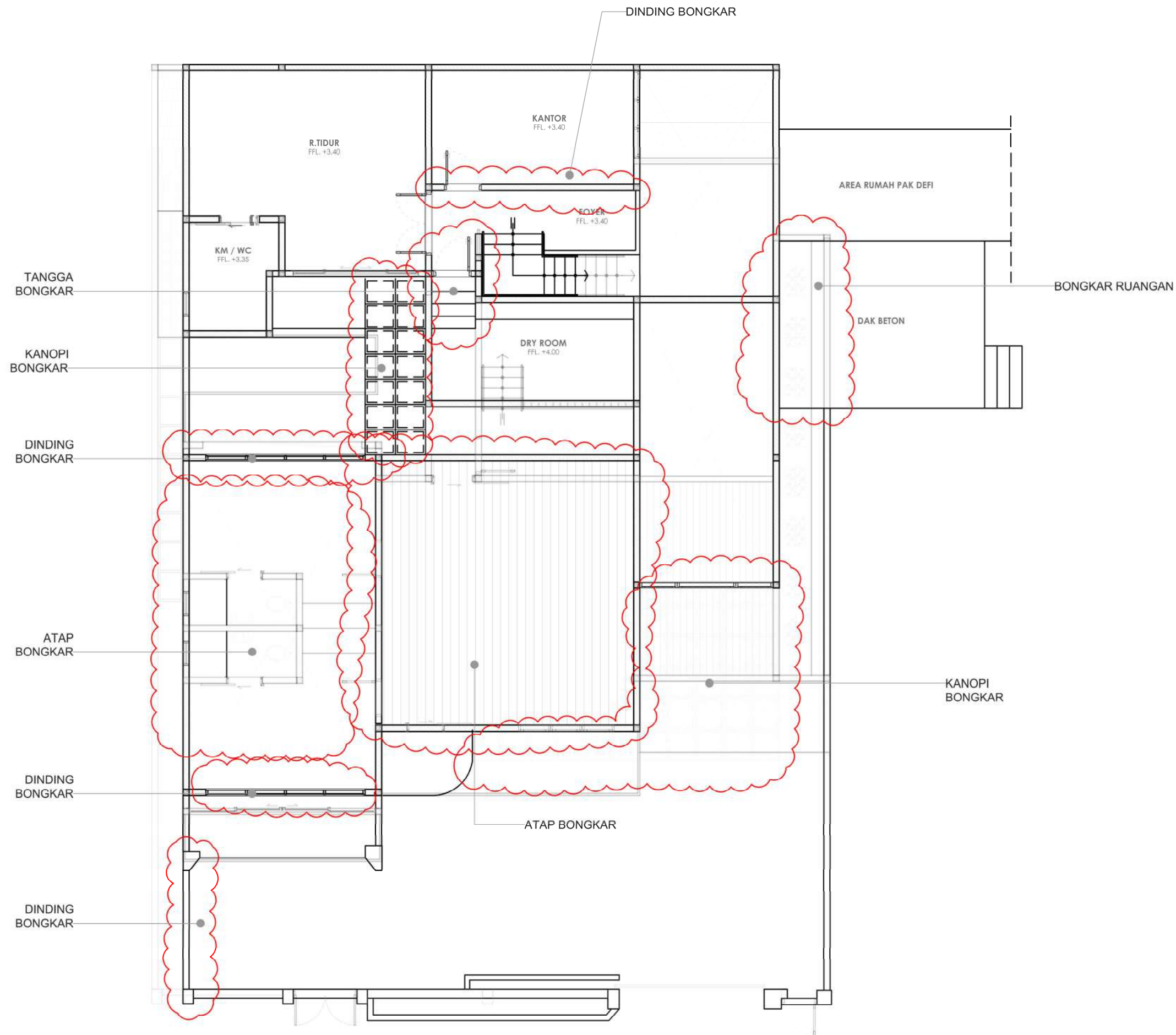
DENAH PEMBONGKARAN LT. 2 SKALA 1:100
