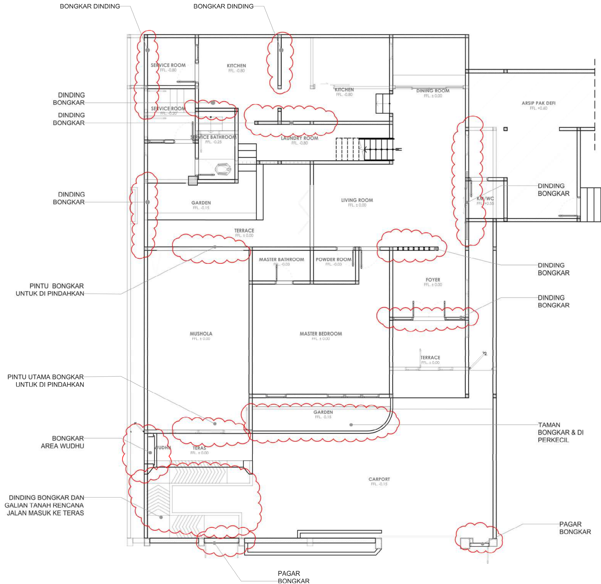
DENAH PEMBONGKARAN LT. 1 SKALA 1:100
