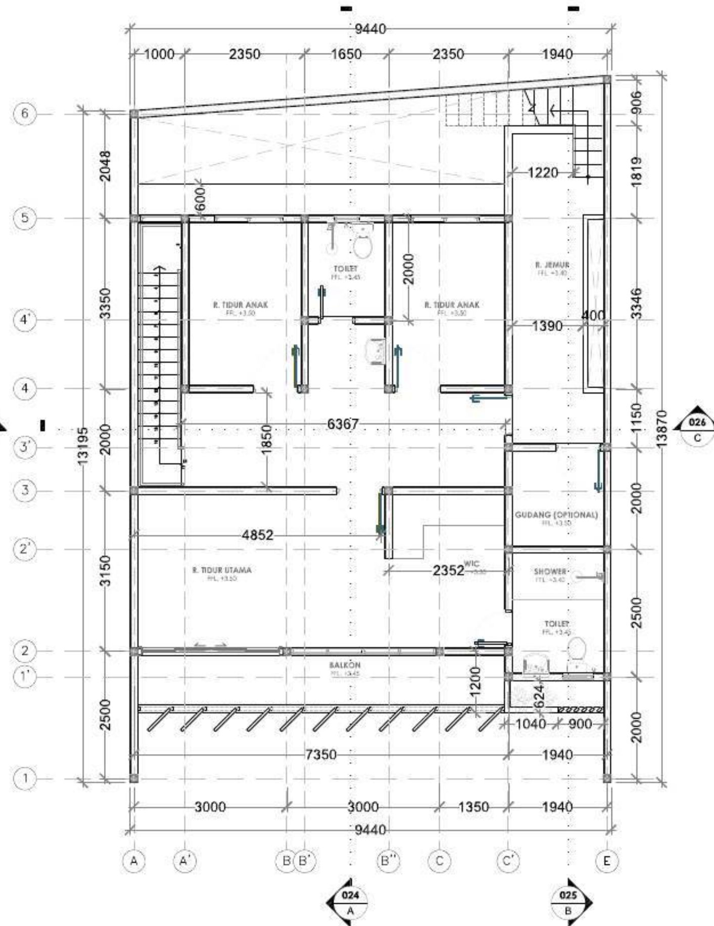
DENAH LANTAI ATAS SKALA 1: 75
