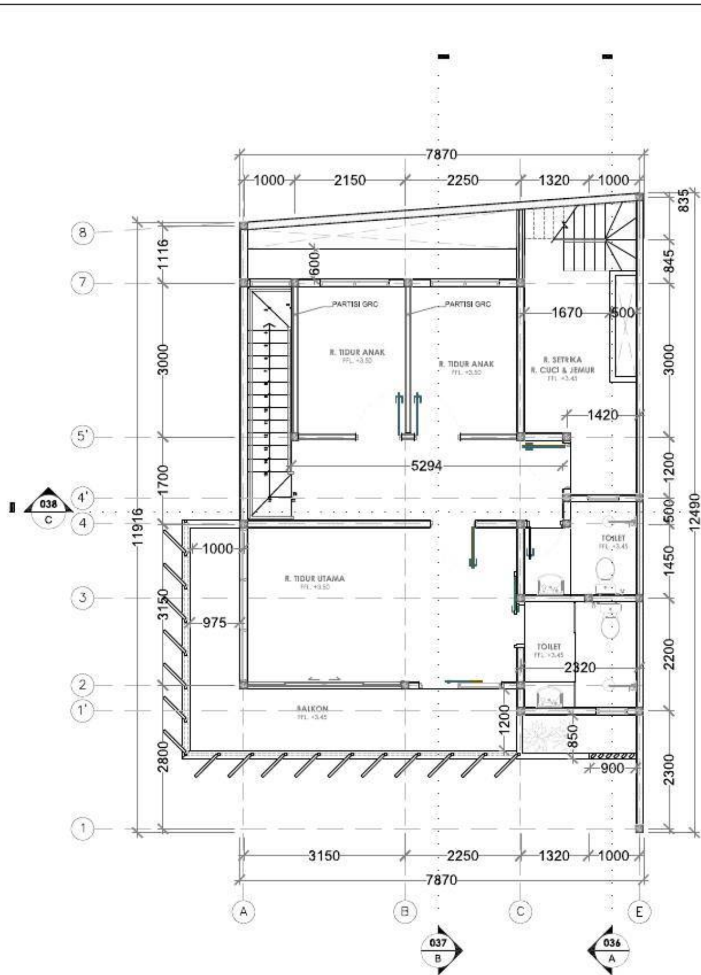
DENAH LANTAI ATAS SKALA 1: 75
