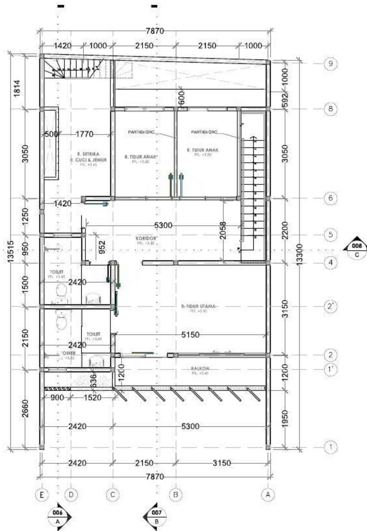
DENAH LANTAI ATAS
