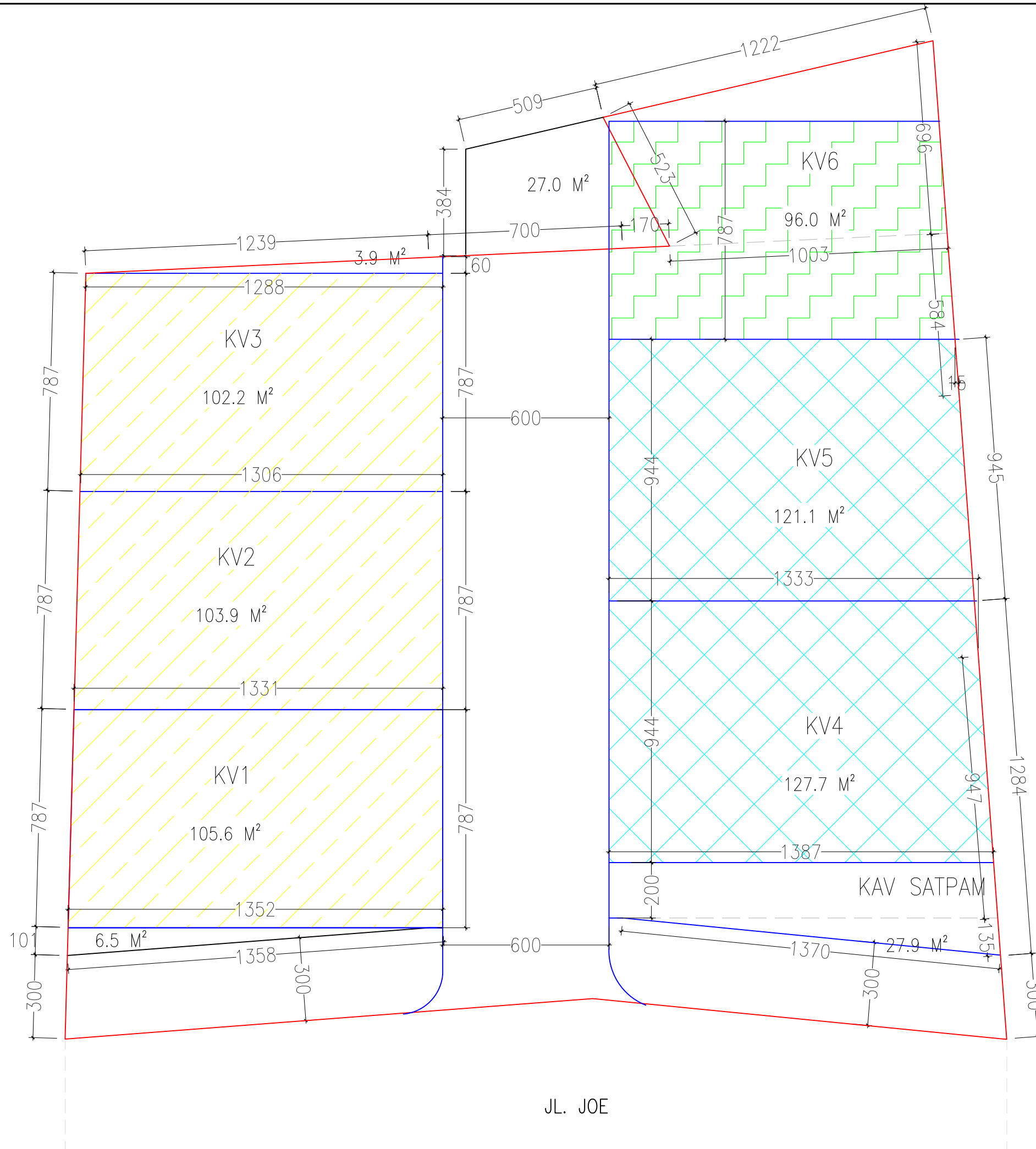
SITE PLAN SKALA 1:150
