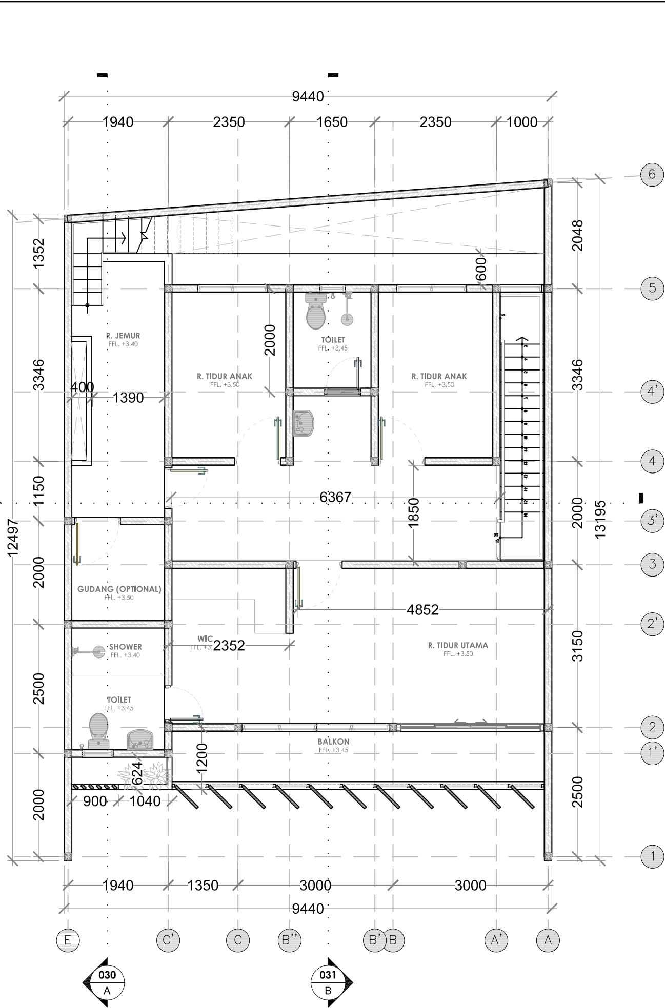
DENAH LANTAI ATAS SKALA 1: 75
