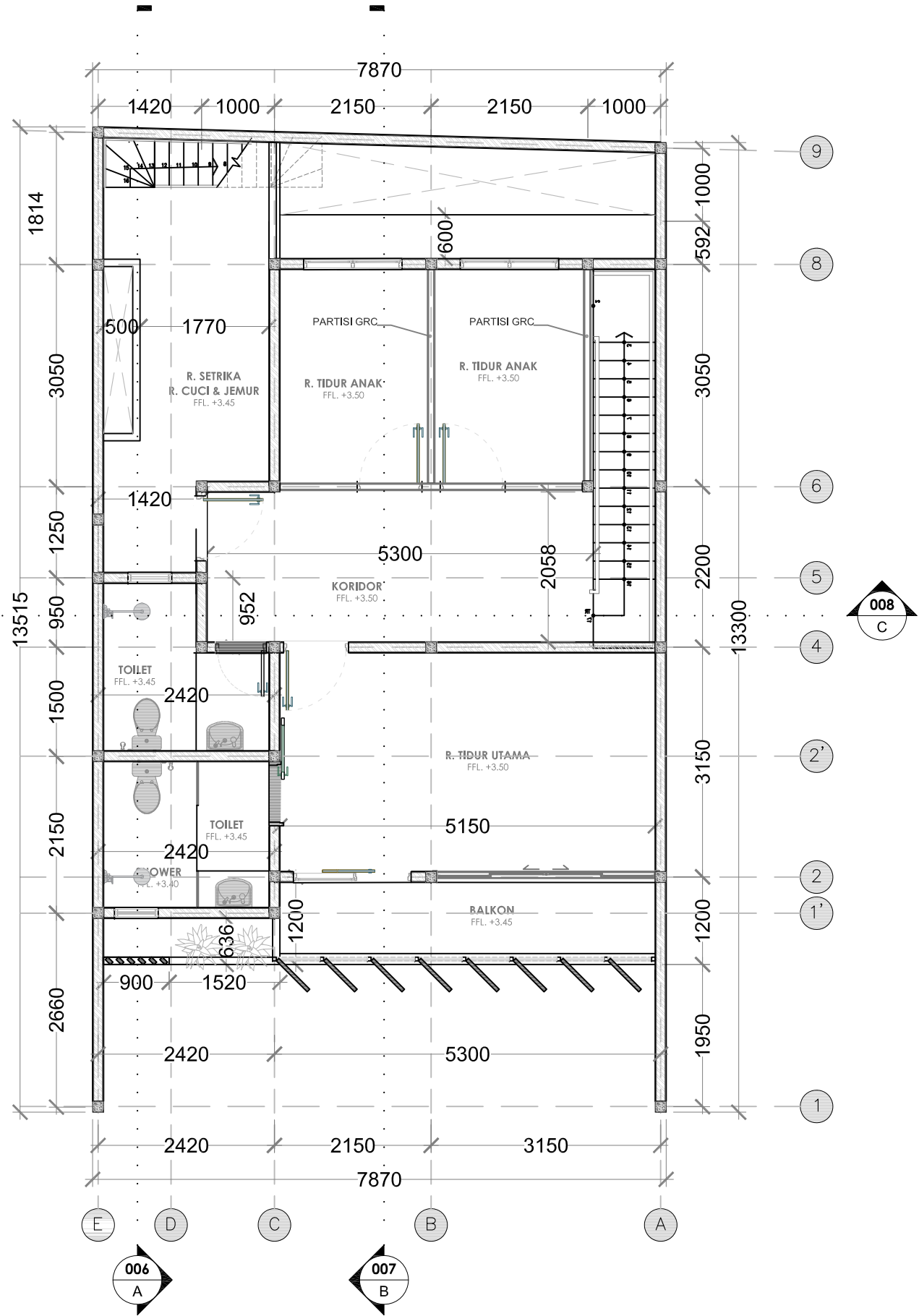
DENAH LANTAI ATAS SKALA 1: 75
