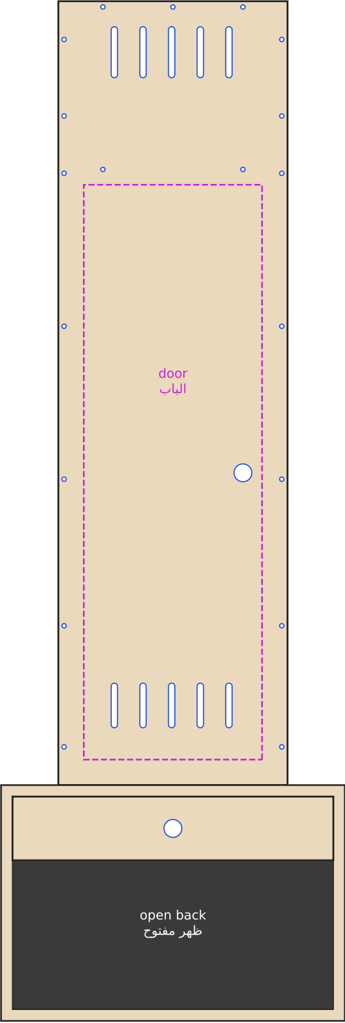
BACK (outside) · الظهر
