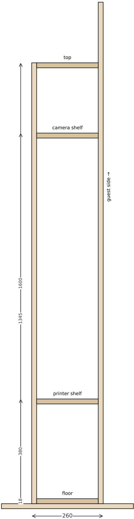
SIDE SECTION · قطاع جانبي
