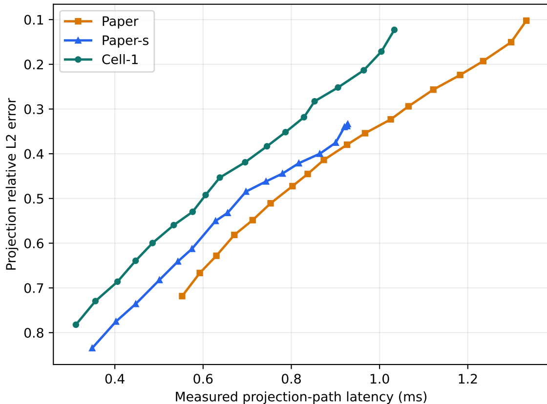
Quality-latency frontier
