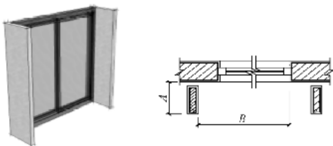
图 B.3.1-2 垂直外遮阳特征值示意图
