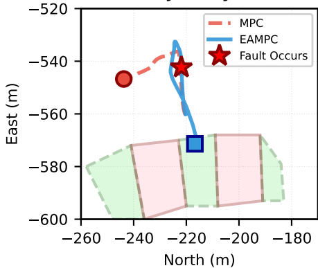
(d) Trajectory (95%)
