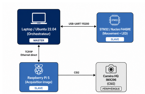
FIGURE 3.2 : Architecture globale du système VisionGuard
