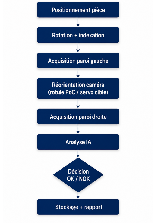
FIGURE 3.1 : Chaîne fonctionnelle du système VisionGuard
