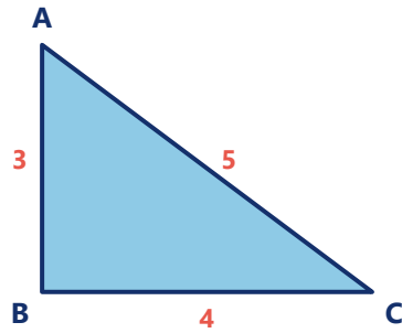
משולש ABC: AB = 3 , CA = 5 , BC = 4
