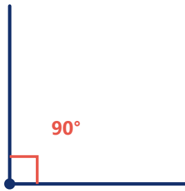
הזווית A — זווית ישרה
