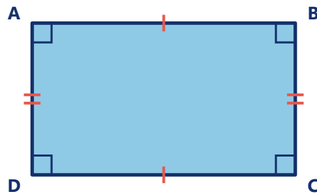
המלבן ABCD — צלעות נגדיות שוות וארבע זוויות ישרות. האלכסון BD אינו מסומן בשרטוט
