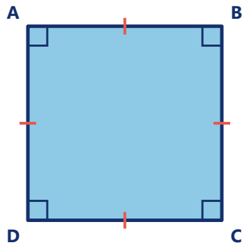
ריבוע ABCD — ארבע צלעות שוות וארבע זוויות ישרות
