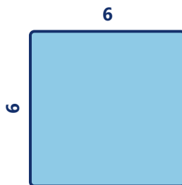
הריבוע שצלעו 6
