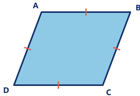
מעוין ABCD — ארבע צלעות שוות, ללא זוויות ישרות
