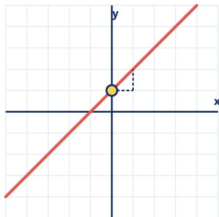
הגרף של y = x + 1
