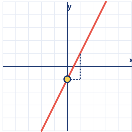
הגרף של y = 2x - 1
