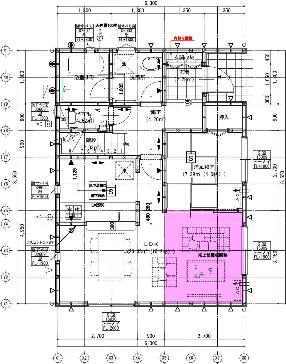
1階 平面詳細図 S:1/75
