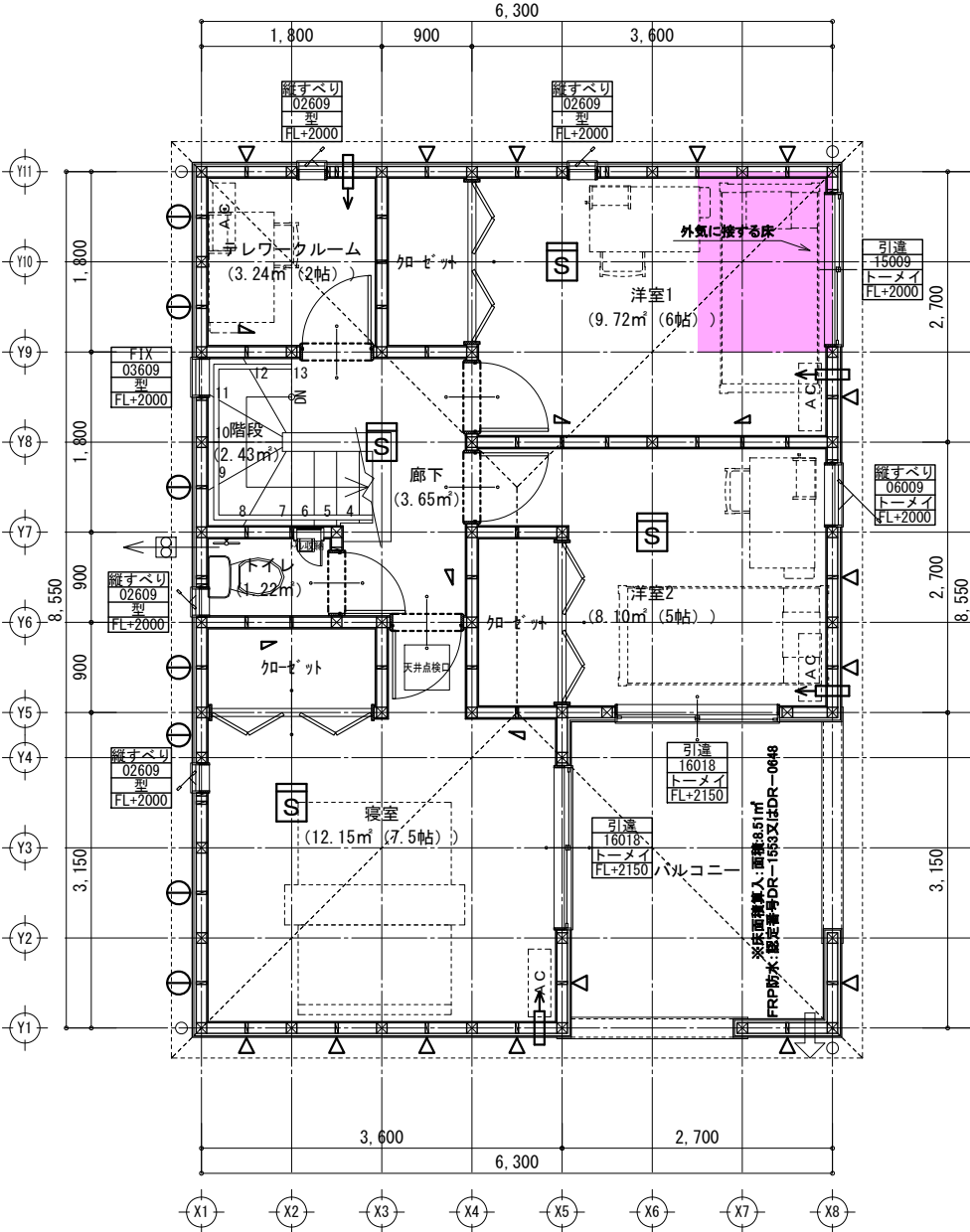
2階 平面詳細図 S:1/75
