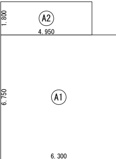
1階 床面積求積図 S:1/200
