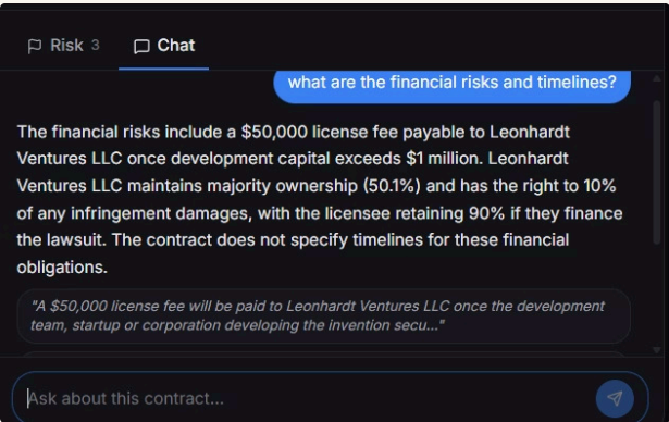
RAG Chat
