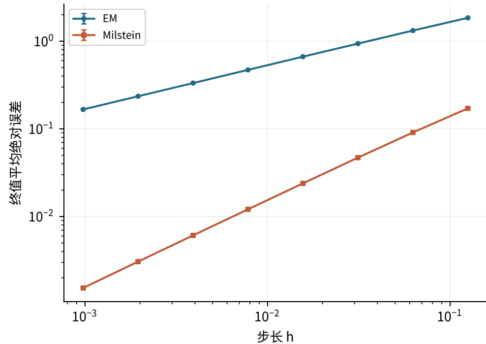
强误差：半阶与一阶
