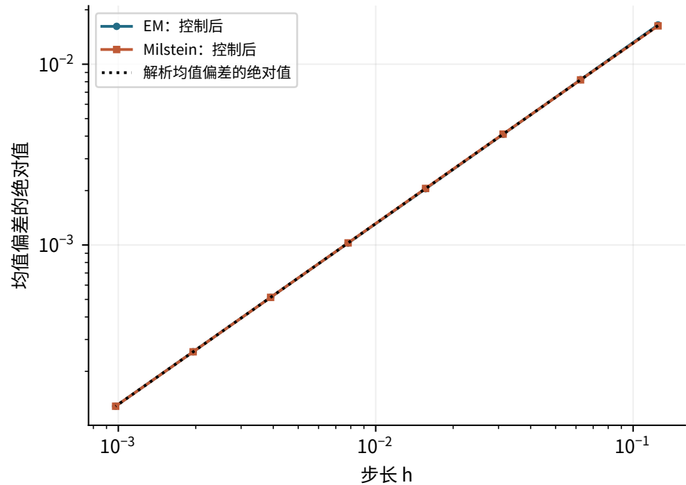
弱偏差：两种方法均为一阶
