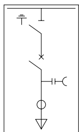
进线柜
