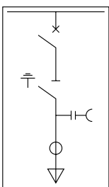
馈线柜
