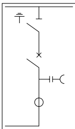
母线进线柜 1
