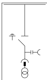
PT 柜
