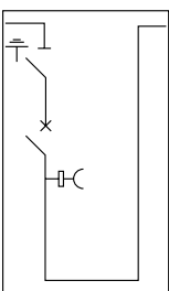
联络柜
