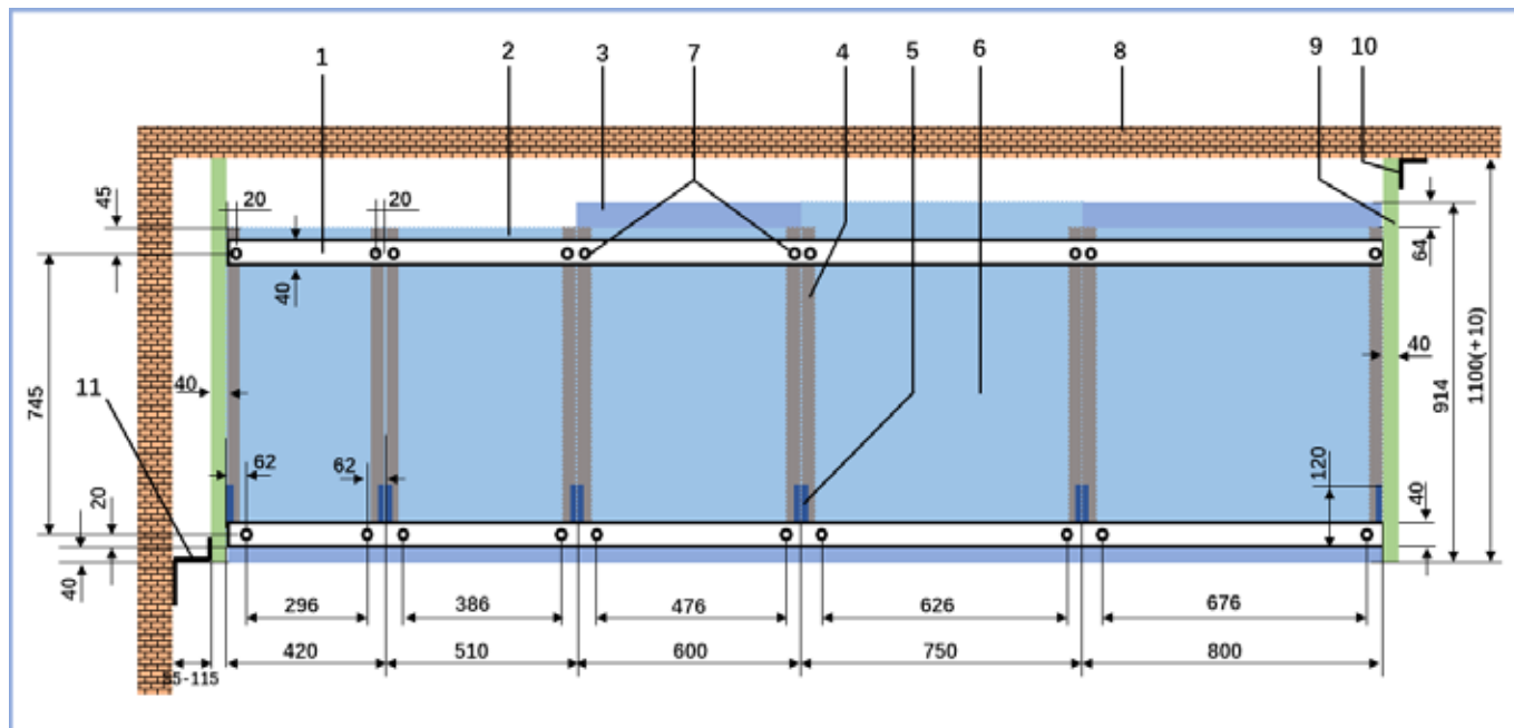
基础槽钢示意图
