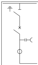
母线进线柜 2
