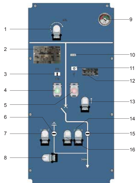
CB-C06 断路器操作面板
