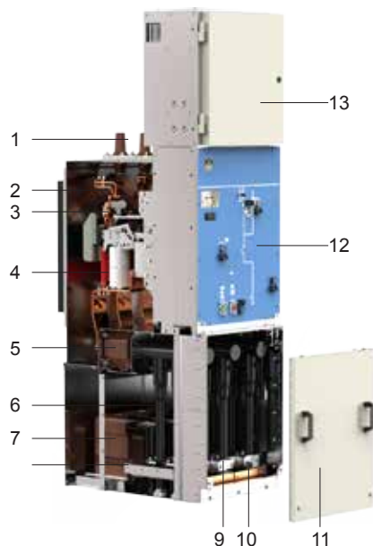
CB-C12 断路器柜
