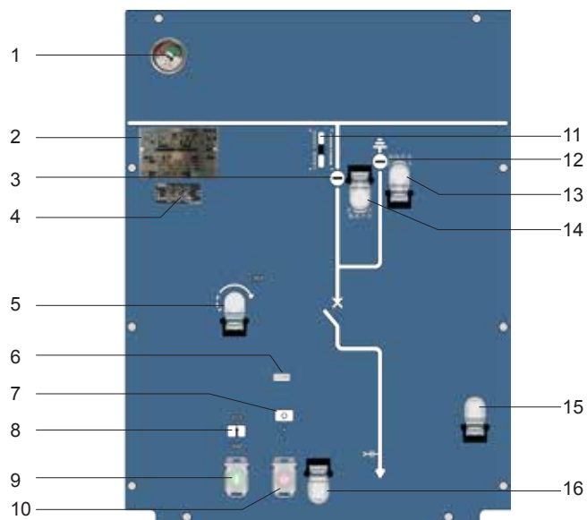
CB-C12 断路器操作面板
