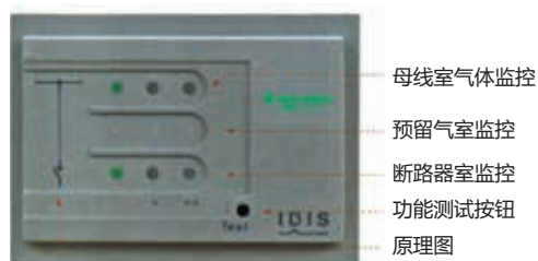
IDIS显示器
