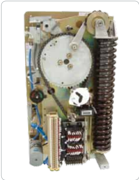
BLRM无外罩操动机构
