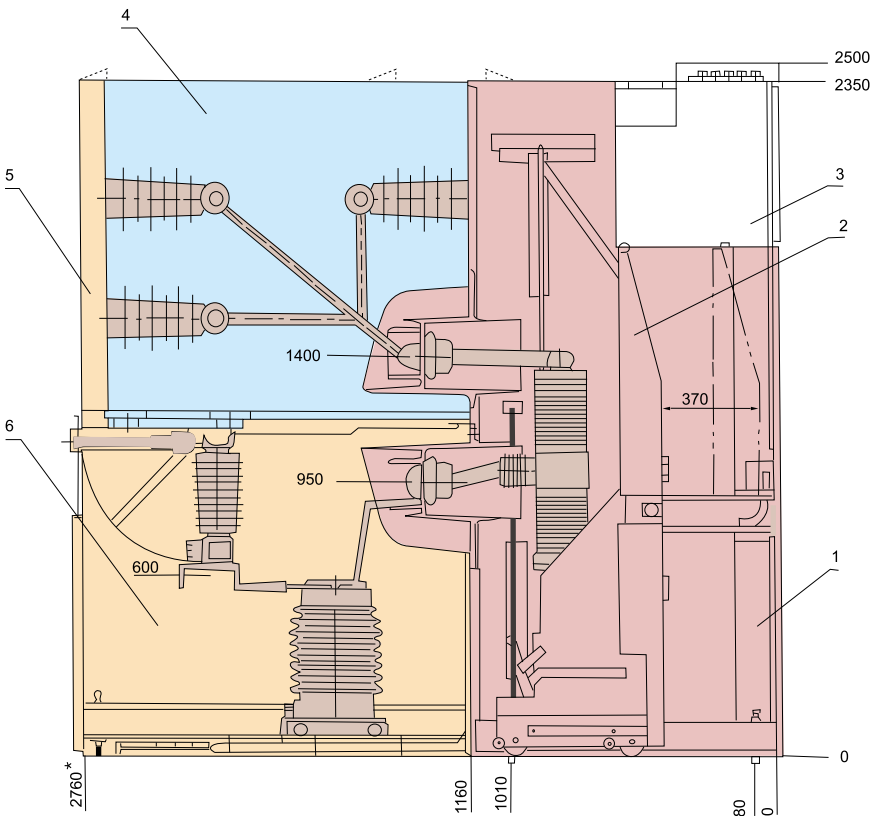
图1、电缆进出线柜内部结构示意图
