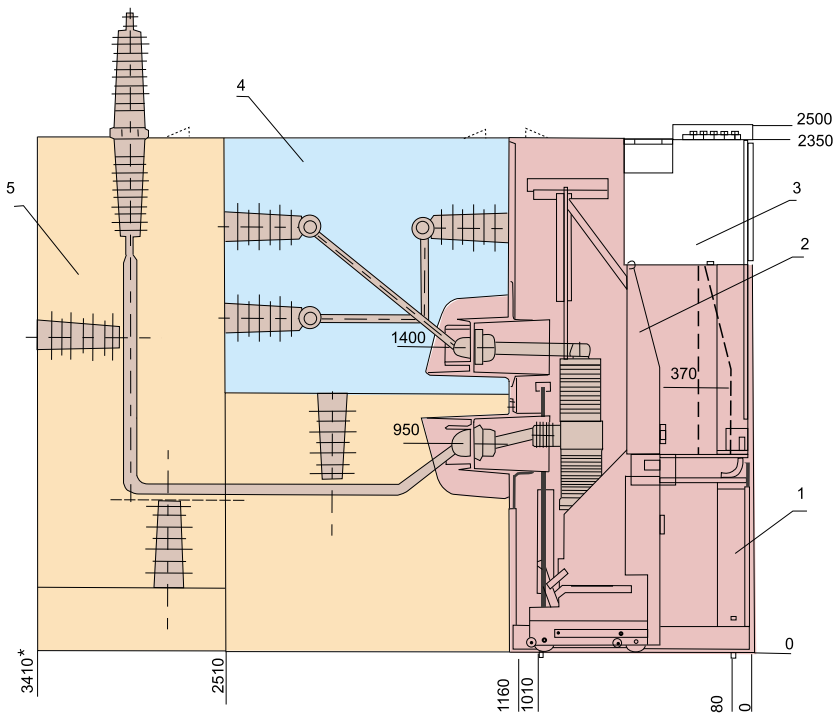
图2、架空进出线柜内部结构示意图
