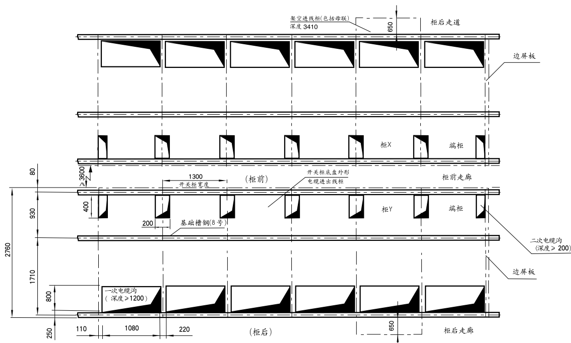
图5 DNF7 基础槽钢埋设示意图(俯视图)
