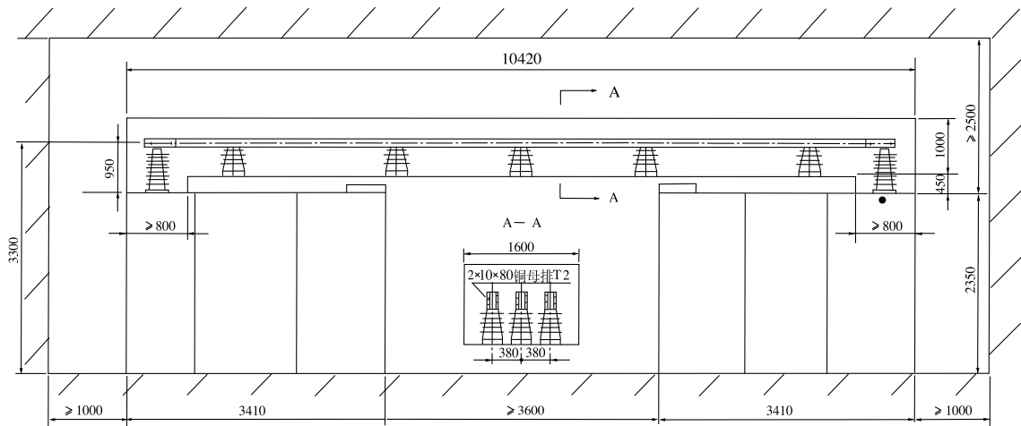
图4 双排列布置图
