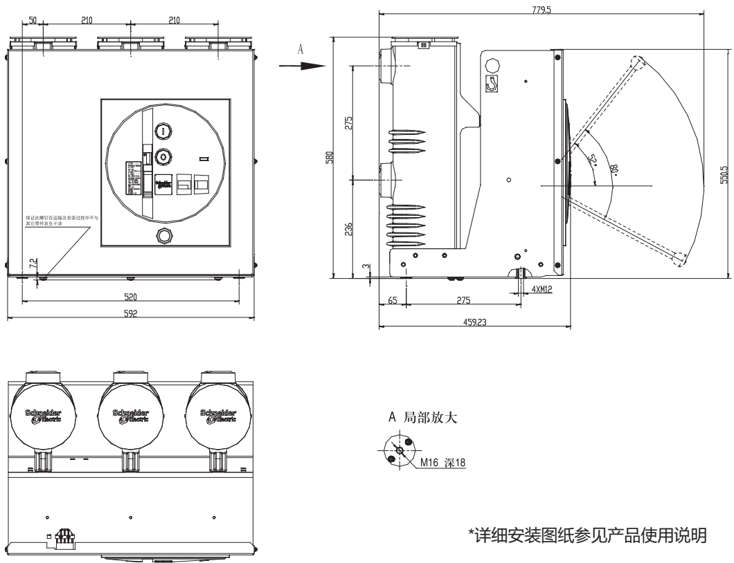
AS12-ES产品 断路器部分相关图纸
