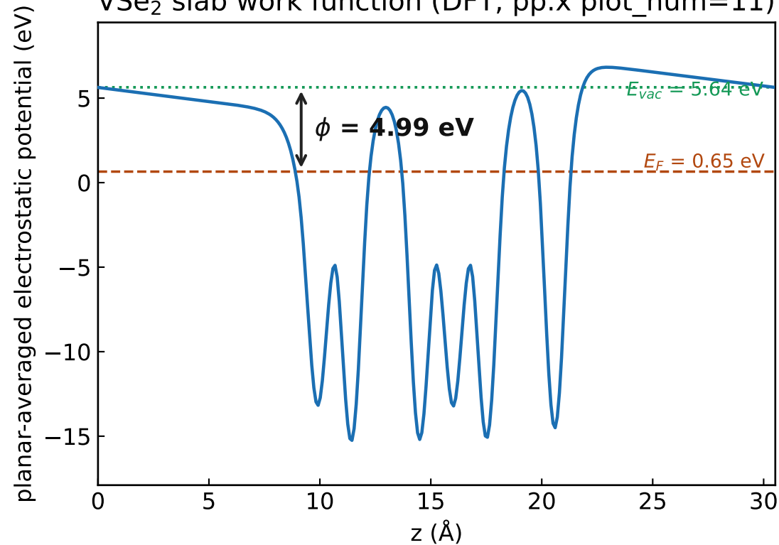
VSe 2 slab work function (DFT, pp.x plot_num=11)
