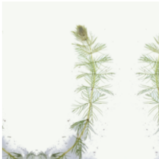
Color Jitter
