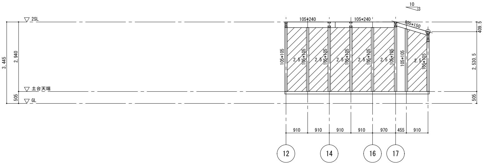
い通軸組図 1/100
