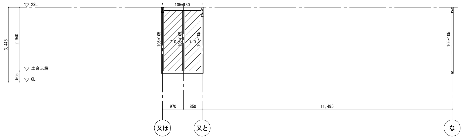
10' 通軸組図 1/100
