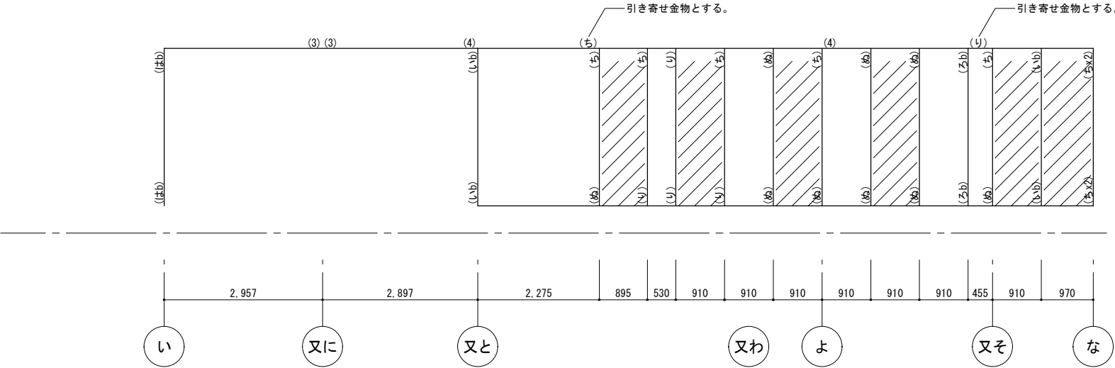
17通軸組図 1/100
