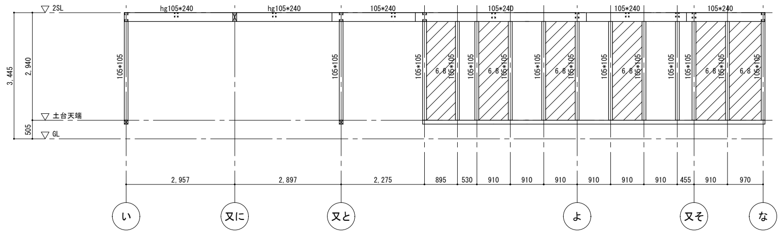
17通軸組図 1/100
