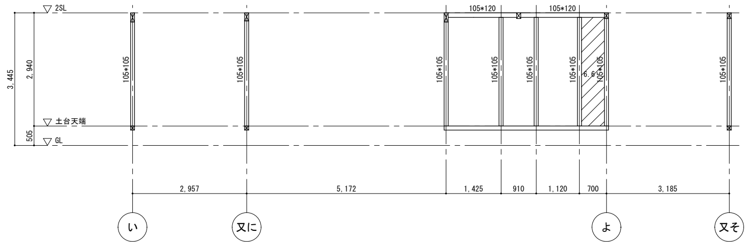
16通軸組図 1/100
