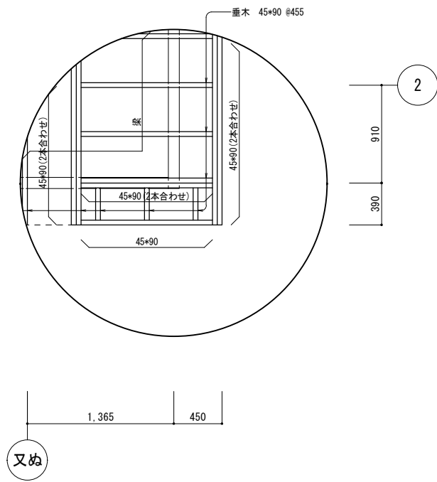
軒先部詳細図B 1/50
