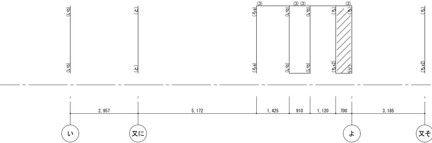
16通軸組図 1/100
