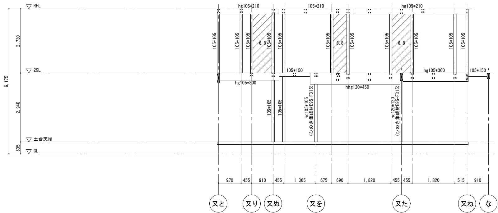
10'' 通軸組図 1/100
