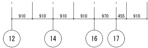
い通軸組図 1/100
