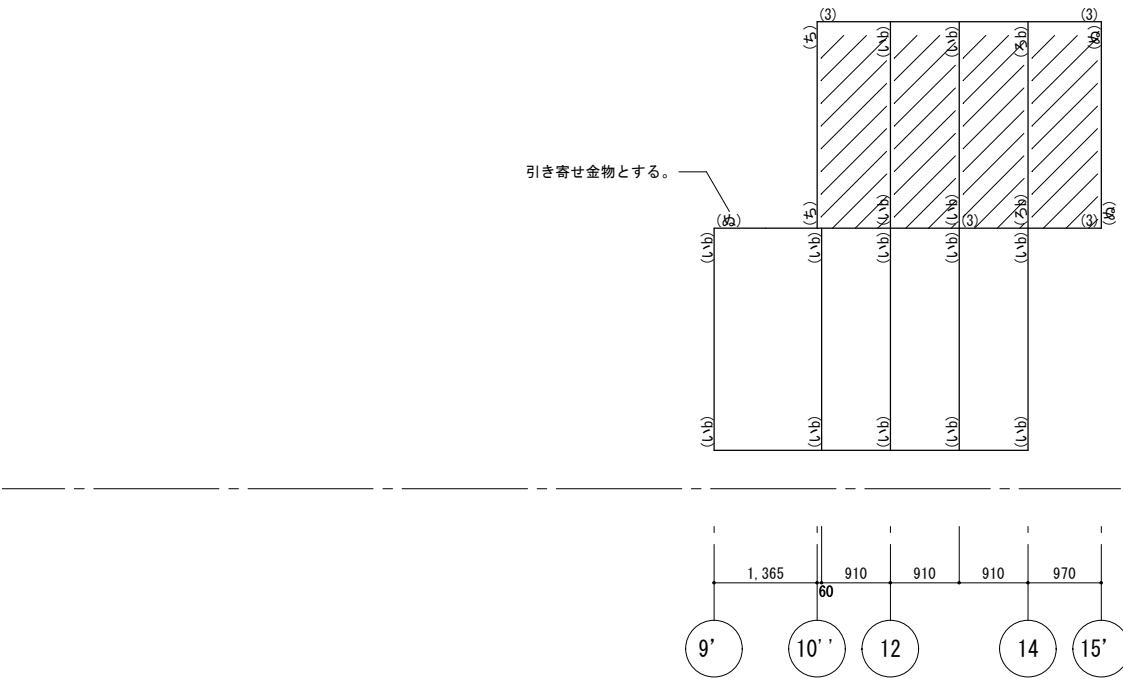
又ね通軸組図 1/100
