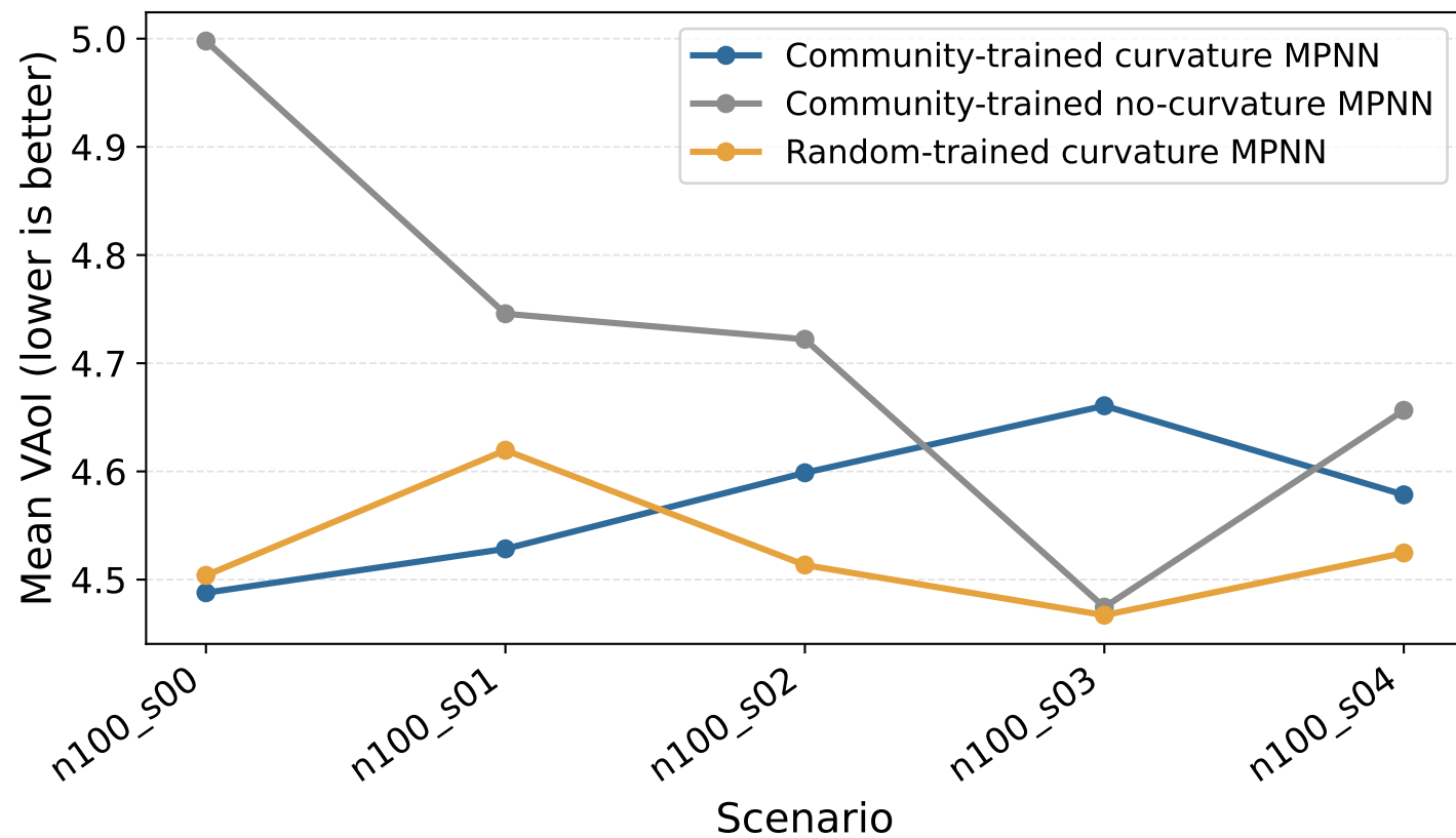
Paired random N=100 scenarios
