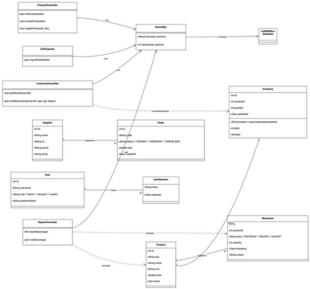
Diagrama de Clases (Actual)
