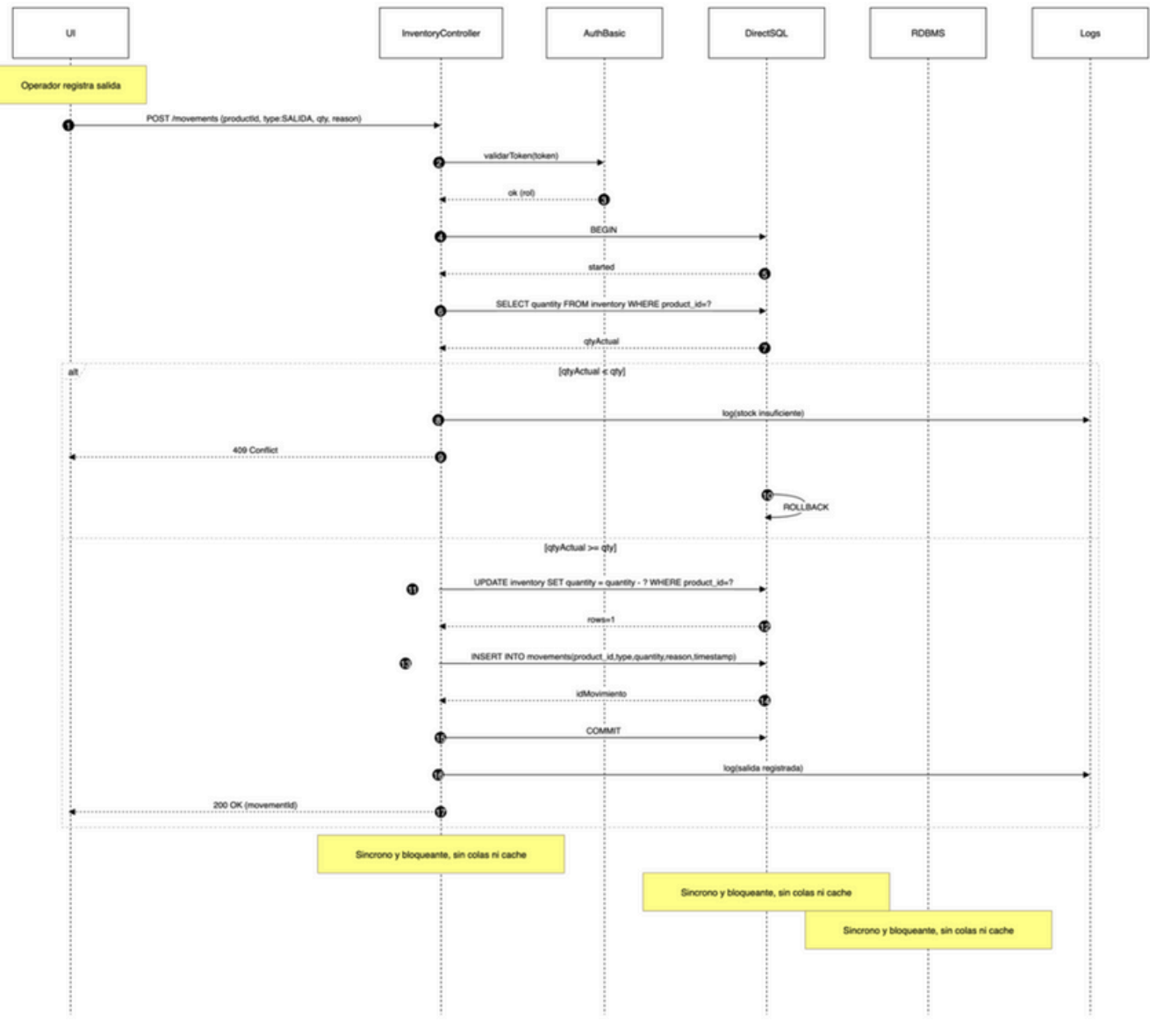
Diagrama de Secuencia (Actual)
