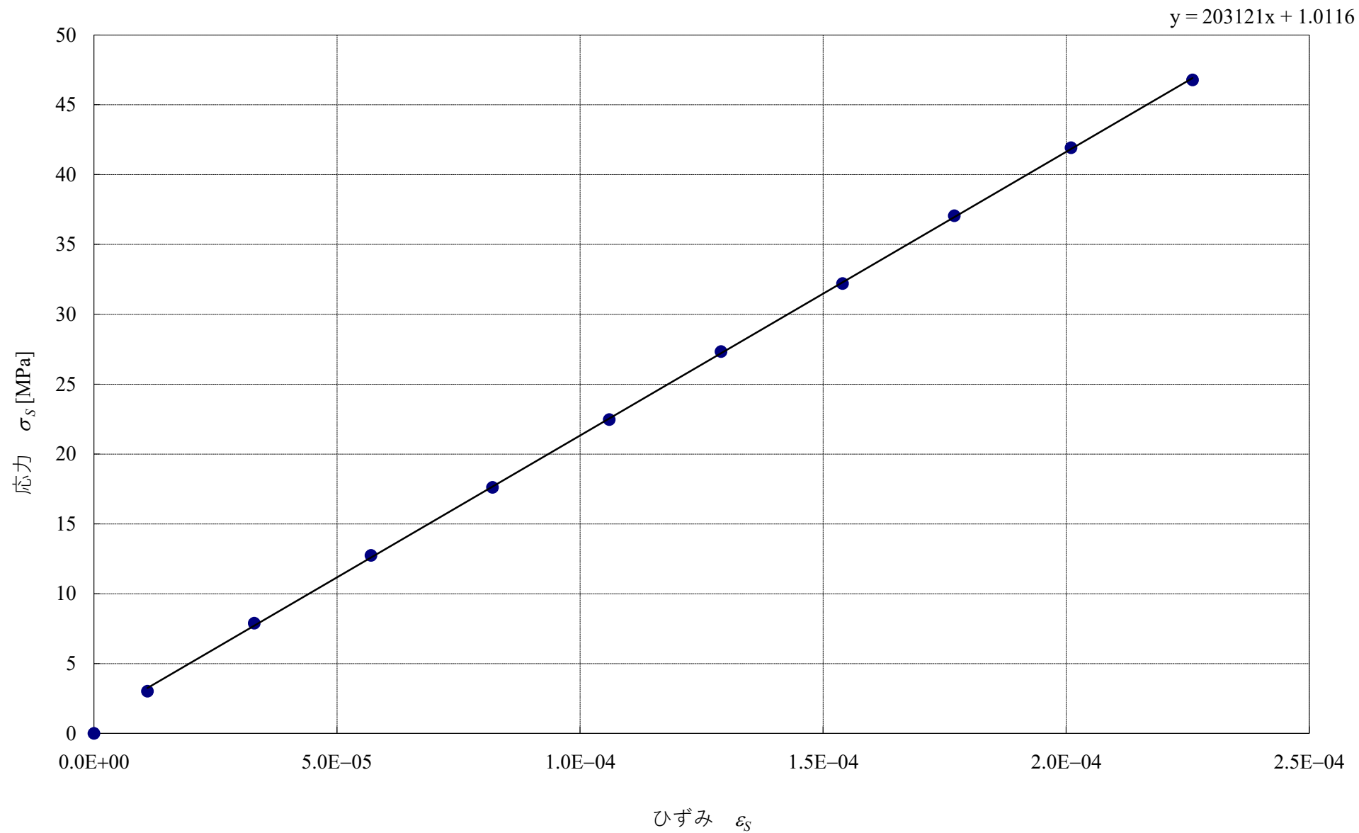
はりのたわみ試験 応力-ひずみ線図
