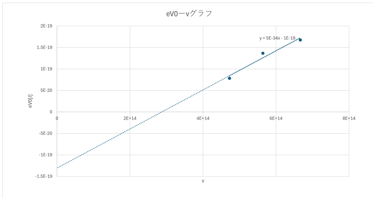
図2 eV 0 -νグラフと回帰直線
