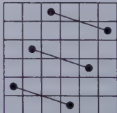
Not a Costas array
