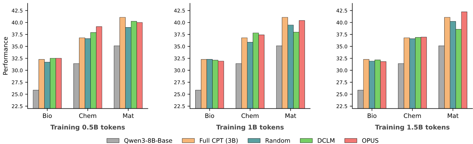
(b) SciAssess
