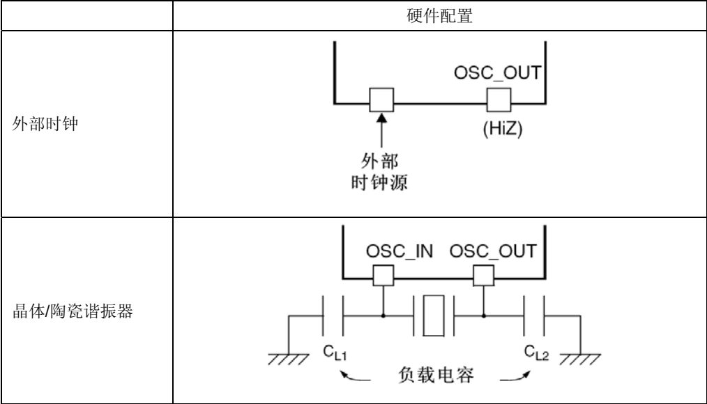
图12 HSE/LSE时钟源
