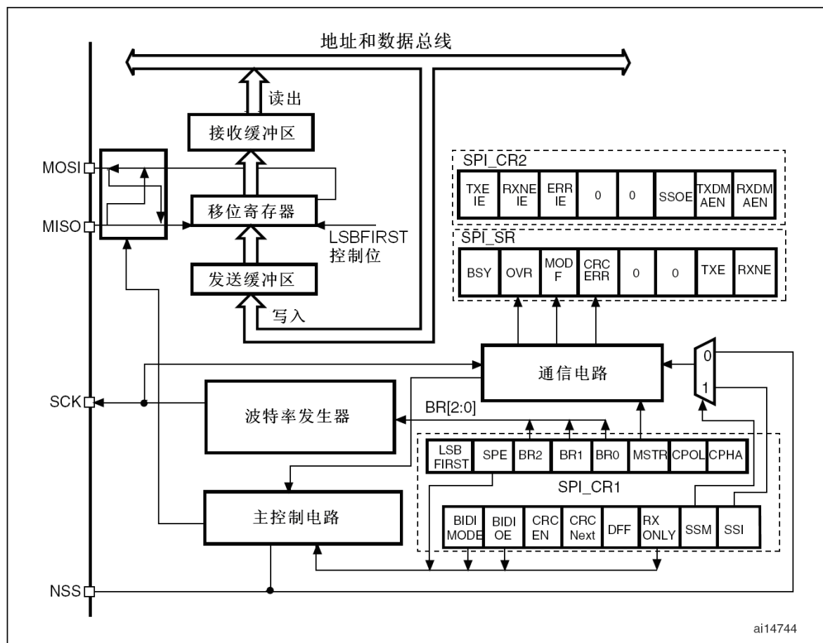
图209 SPI框图
