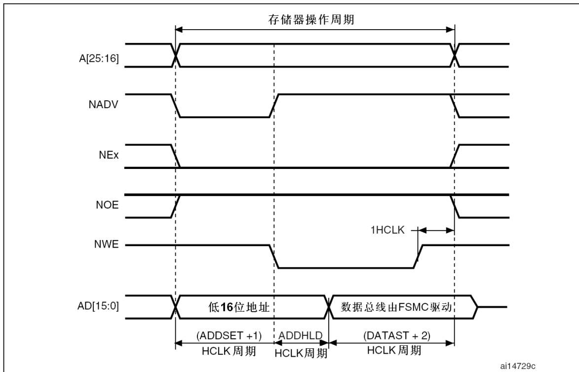
图174 复用写操作
