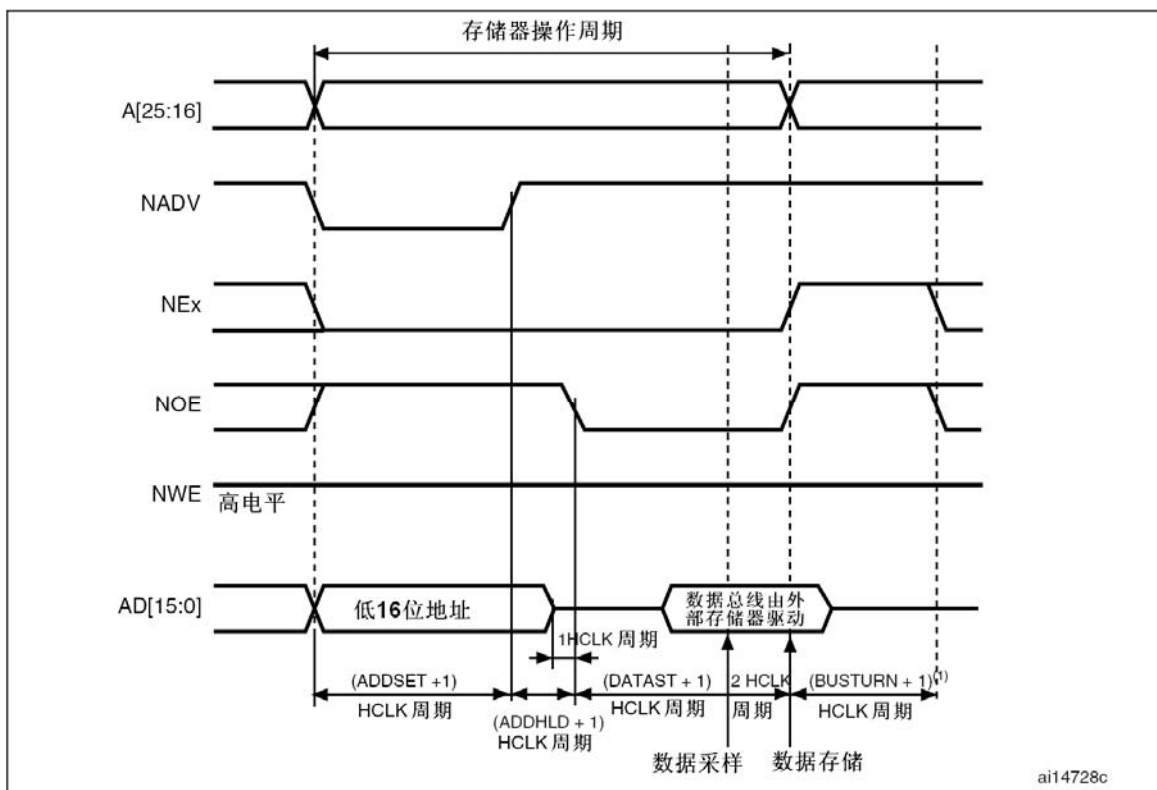
图173 复用读操作
