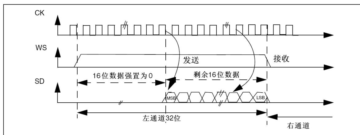
图235 LSB对齐16位数据扩展到32位包帧，CPOL = 0
