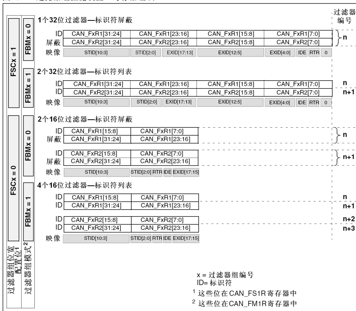
图202 过滤器组位宽设置一寄存器组织
