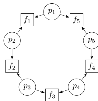
(a) Graf filozofa
