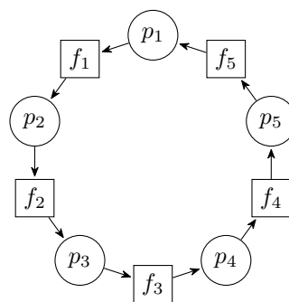
(b) Deadlock filozofa
