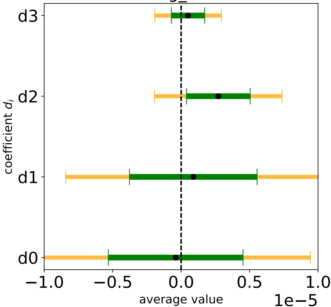
config_40 1K
