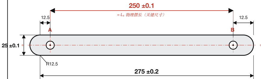
前视图 Front View (2:1 显示)
