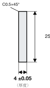
侧视图 Side View (5:1 放大) 孔位详图 Hole Detail (8:1, A、B 通用)
