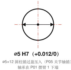
孔 A 详图 (8:1) · \phi 5 H7
