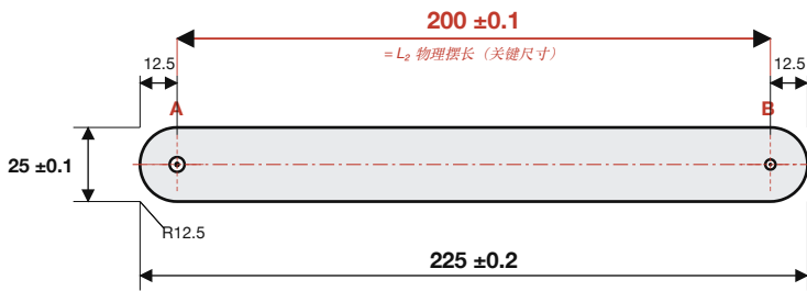
前视图 Front View (2:1 显示)
