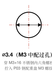
孔 B 详图 (10:1) · M3 通孔
