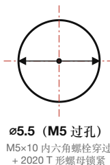
轴孔 S 详图 Shaft Hole Detail (8M5 安装孔详图 (8:1))
