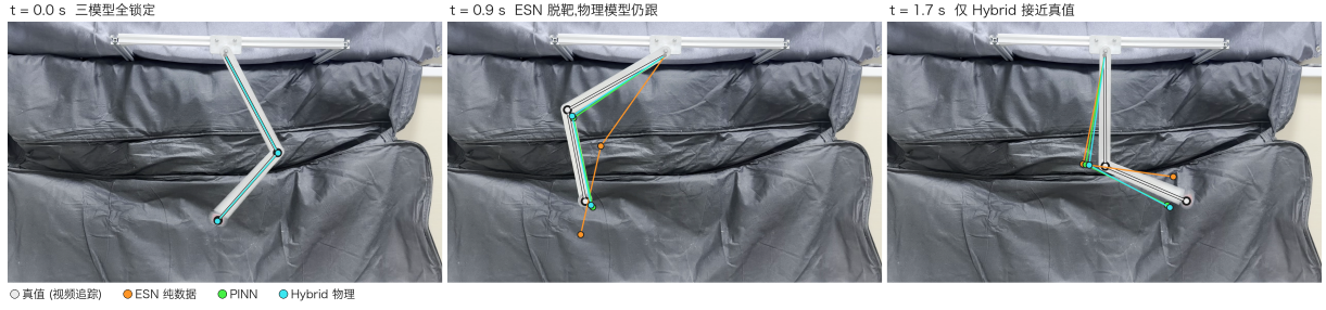
图 5: 真实录像上的零样本预测叠加 (IMG_1448, 释放角 66^\circ )。黑色描边的白线为视频追踪真值, 橙/绿/青分别为 ESN/PINN/Hybrid 从视频反演初值出发的闭环预测, 逐帧投影回像素平面。 t = 0 三模型与真值重合; t = 0.9\text{s} 数据驱动 ESN 已脱靶而物理先验模型仍贴合; t = 1.7\text{s} 仅 Hybrid 接近真值——物理结构在真实数据上把可信预测窗口延长数倍, 与表 3 一致。
