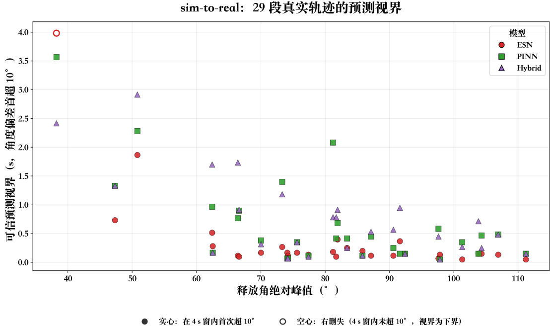
图 6: 29 段真实轨迹上三方视界随释放角的分布。实心标记表示在 4s 窗内首次达到 10^\circ 偏差; 空心标记为右删失 (窗口内未达阈值, 取窗长为视界下界)。
