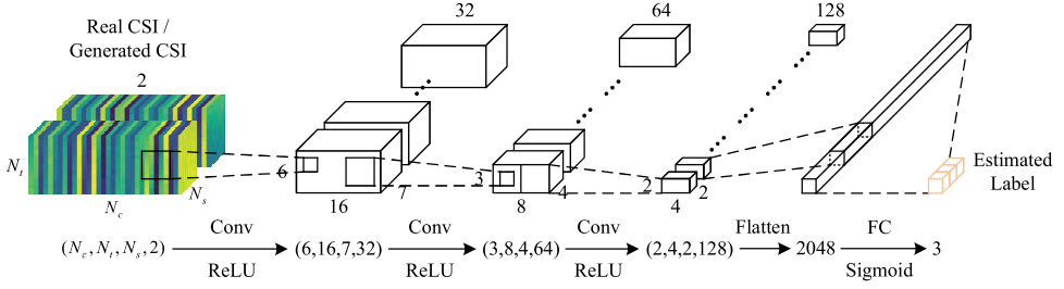
(a) Estimator
