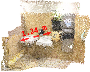
Ours
