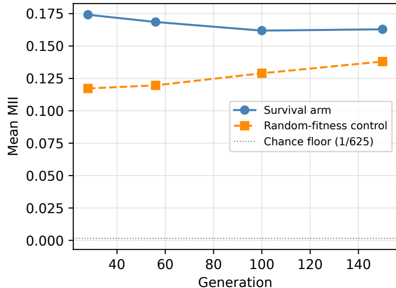
MII trajectories (n=24)
