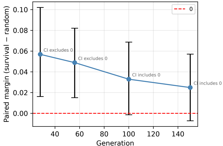
Margin trajectory (n=24, 95% CI)
