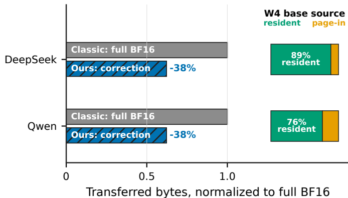
(d) Correction traffic reuses resident W4
