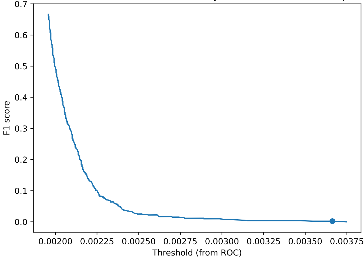
Mink r=1.0 — F1 vs Threshold (best by ROC: max TPR - FPR, skip inf)
