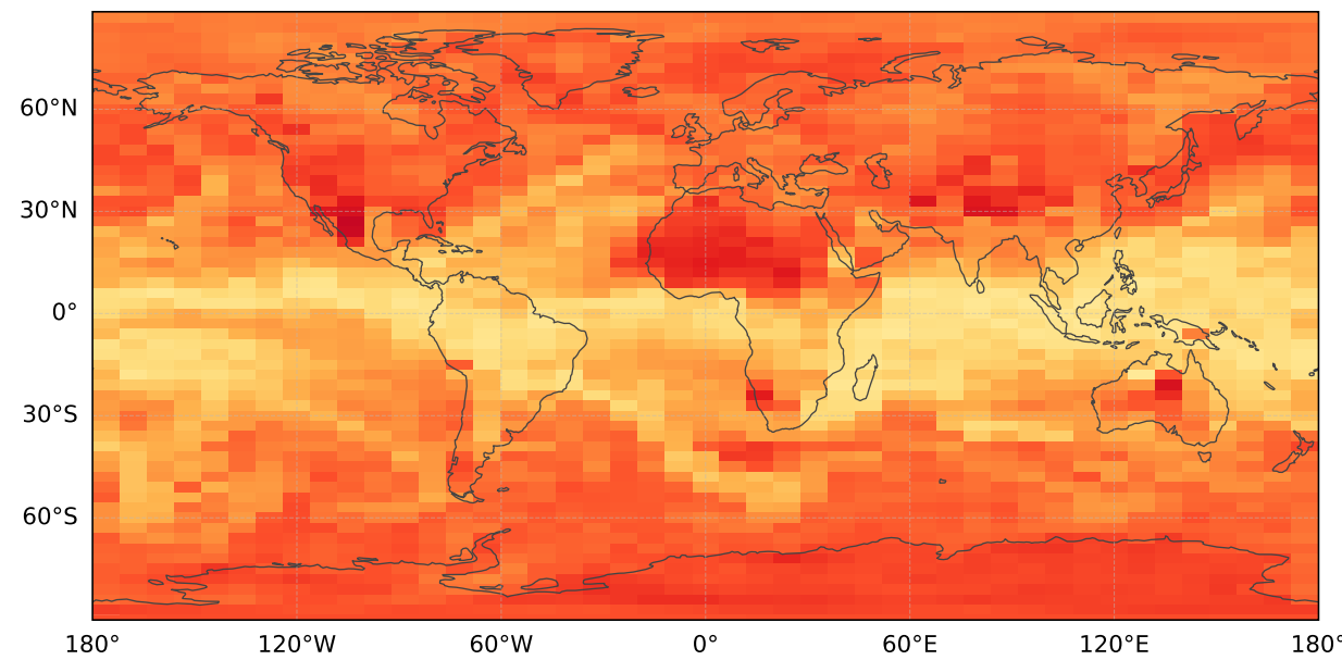
(d) \partial F_{\text{OLR}}/\partial T_{\text{sfc}}
