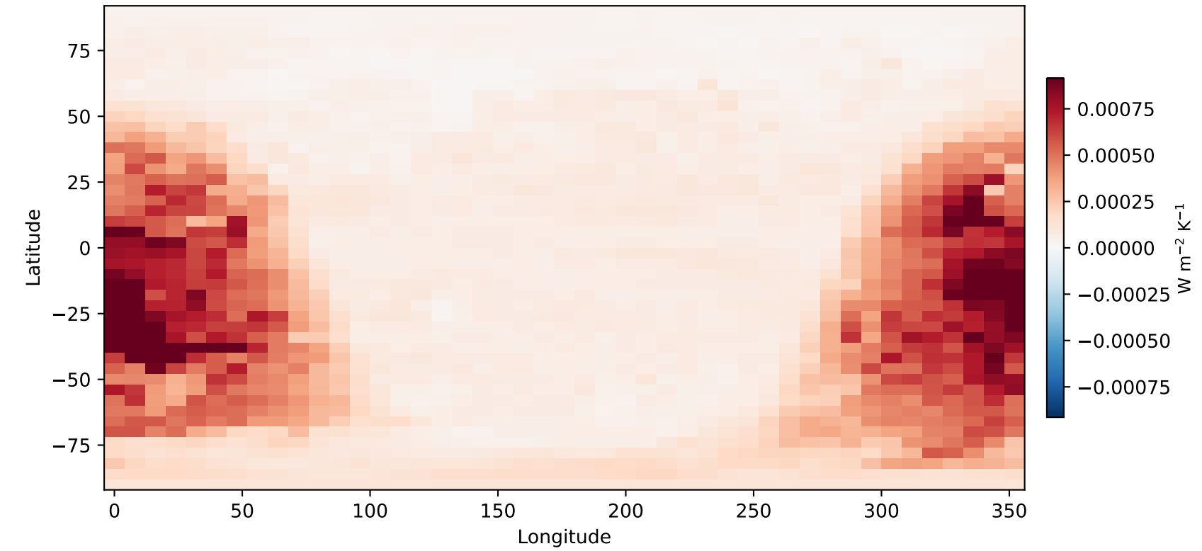
(d) \partial F_{\text{sfc}} / \partial \mu_0
