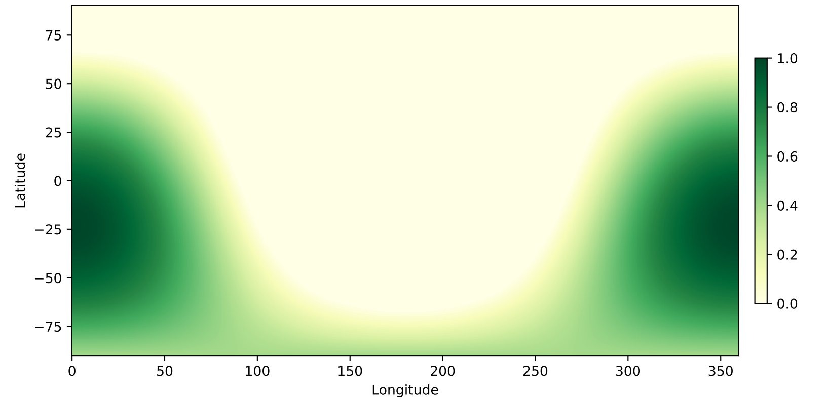
(d) Cosine Solar Zenith ( \mu_0 )
