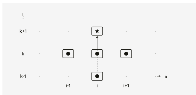
显式差分格式取点示意图（向前差分）
