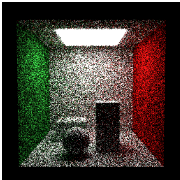
Figura 1. Cornell Box difusa, amostragem por BSDF.
