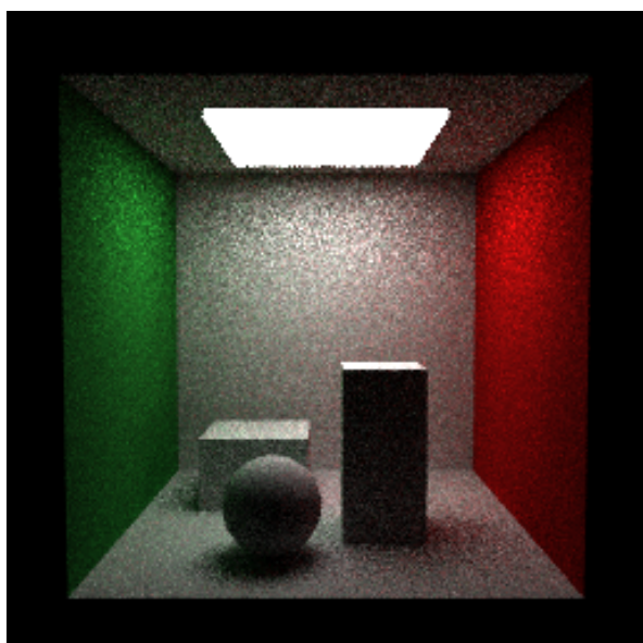
Figura 2. Amostragem direta da luz (NEE): menor variância que BSDF-only no mesmo SPP.
