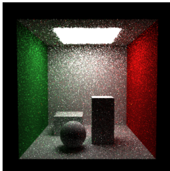
Figura 4. MIS + Roleta Russa: mesma média, menor custo em caminhos profundos.
