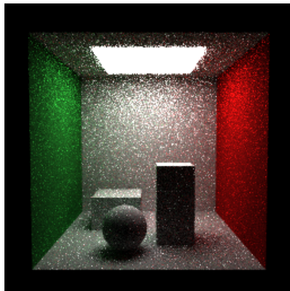
Figura 3. MIS (heurística de potência \beta = 2 ) combinando BSDF e NEE.
