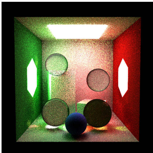
Figura 22. Cena combinada com esfera espelhada, mis (512×512, SPP=4, estratificado, depth=4): combina BSDF e NEE com heurística de potência ( \beta = 2 ); reflexão especular da esfera espelhada bem definida; menor variação nas superfícies difusas; regiões TIR visíveis nas esferas dielétricas.
