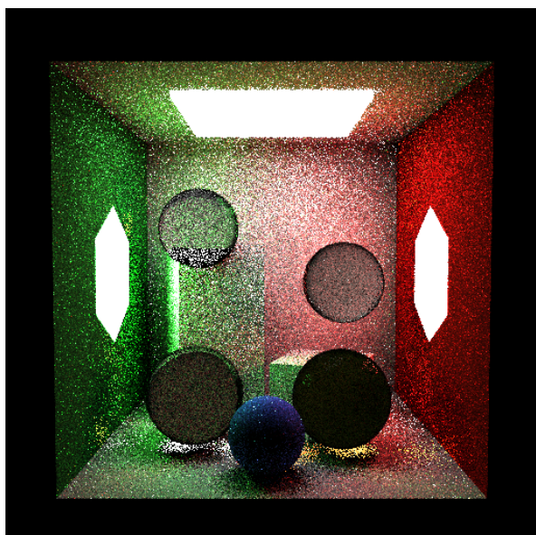
Figura 23. Cena combinada com esfera espelhada, mis + Roleta Russa (512×512, SPP=4, estratificado, depth=4): terminação probabilística de caminhos de baixo throughput ; esfera espelhada reflete múltiplas fontes com redução de tempo de render mantendo estimador não-viesado.
