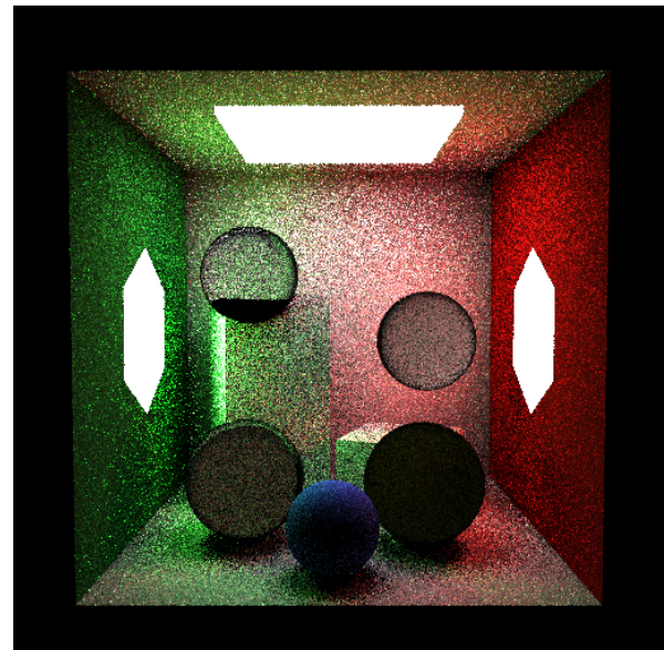
Figura 21. Cena combinada com esfera espelhada, nee_only (512×512, SPP=4, estratificado, depth=4): iluminação direta das três fontes nítida nas superfícies difusas; esfera espelhada e dielétricas especulares ainda ruidosas pois NEE é pulado em bounces dielétricos ( is_specular ).
