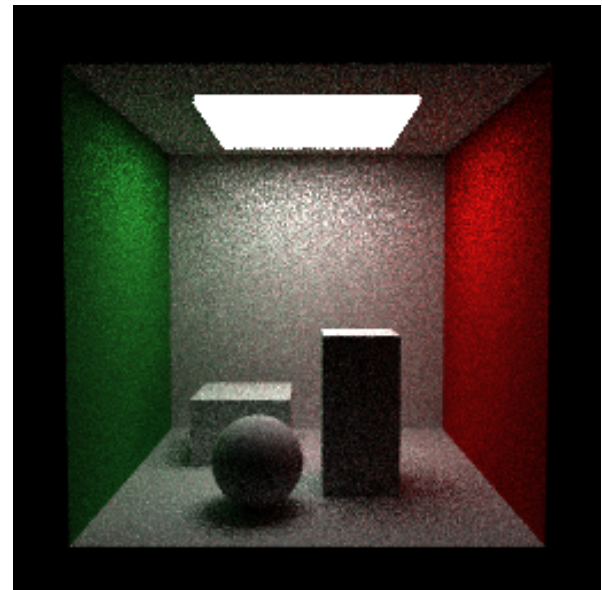
Figura 2. NEE — execução 1 (256×256, SPP=16, seed=42, \approx 1.89 min): amostragem direta da luz, menor variância que BSDF-only.
