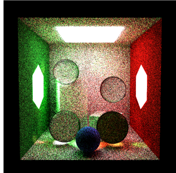
Figura 20. Cena combinada com esfera espelhada, bsdf_only (512×512, SPP=4, estratificado, depth=4): alta variância; reflexões especulares da esfera espelhada amostradas raramente via BSDF puro; esferas dielétricas com regiões escuras por depth esgotado.
