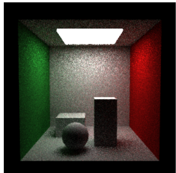
Figura 3. NEE — execução 2 (256×256, SPP=16, seed=42, \approx 1.99 min): consistência entre runs demonstra reprodutibilidade do estimador.
