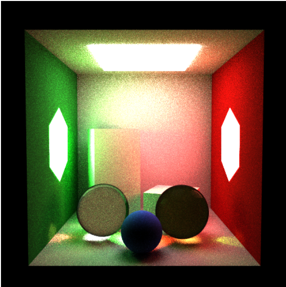
Figura 16. Showcase — mis (512×512, SPP=64, estratificado, depth=12, ≈102 min): combina BSDF e NEE com heurística de potência ( \beta = 2 ); menor variância em superfícies difusas e especulares.
