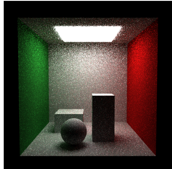
Figura 7. MIS + RR com profundidade mínima 4 (512×512, SPP=12, ≈7,5 min), gerado com --use-rr 4 : maior resolução evidencia a uniformidade da convergência.
