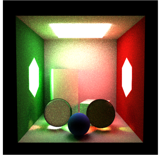
Figura 17. Showcase — mis + Roleta Russa (512×512, SPP=64, estratificado, depth=12, ≈70 min): mesma média, terminação probabilística de caminhos profundos.
