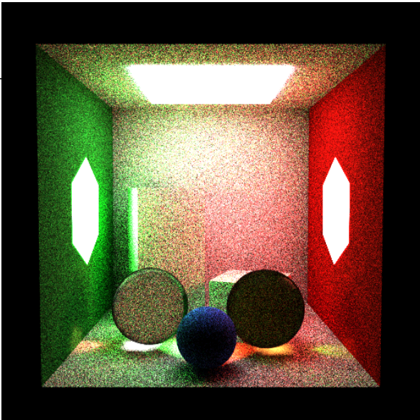
Figura 14. Showcase — bsdf_only (512×512, SPP=64, estratificado, depth=12, ≈42 min): alta variância; as fontes hexagonais laterais são raramente amostradas por BSDF puro.
