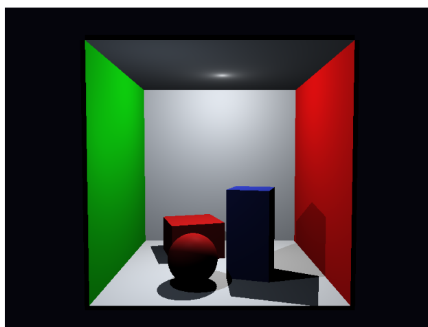
Figura 4. Cena de sombreamento local com Phong e sombras diretas duras por visibilidade até a fonte (800x600, spp=1).
