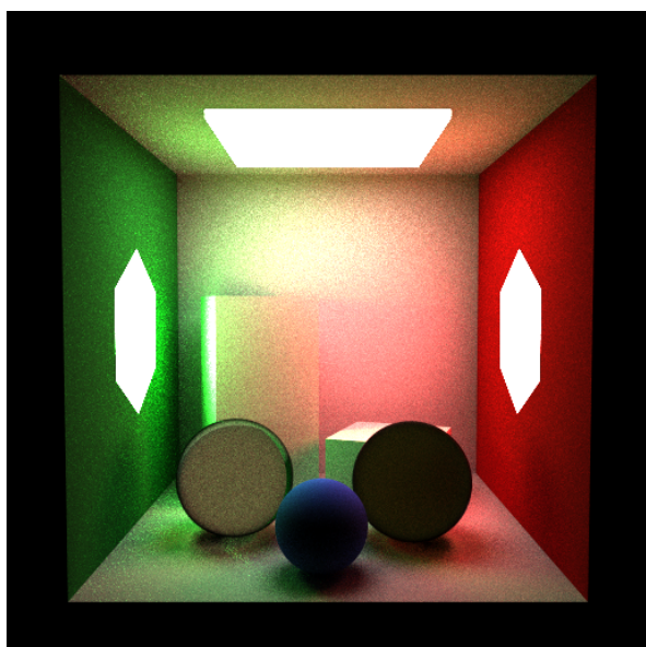
Figura 14. Wall lights — nee_only : amostragem direta das três fontes (teto + paredes); iluminação direta nítida.
