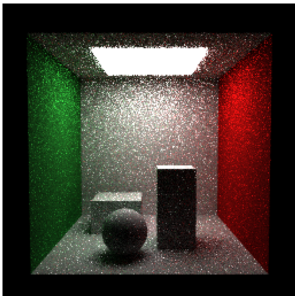
Figura 4. MIS sem Roleta Russa (256×256, SPP=16, seed=42): referência de variância para comparação.
