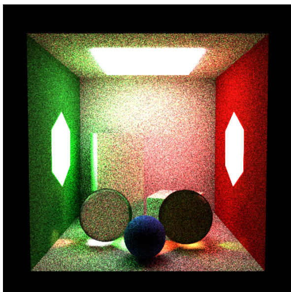
Figura 13. Wall lights — bsdf_only : alta variância pois as fontes hexagonais laterais são raramente amostradas por BSDF.
