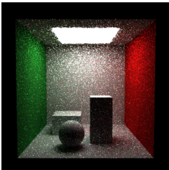
Figura 5. MIS com Roleta Russa (256×256, SPP=16, seed=42): mesma média, menor custo em caminhos profundos.
