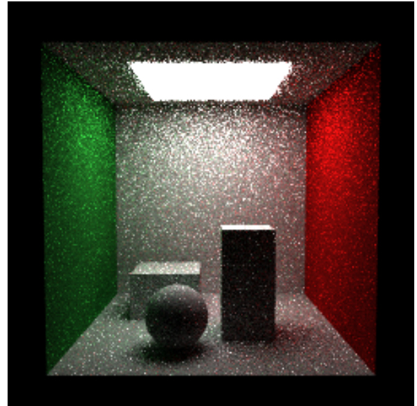
Figura 3. MIS (heurística de potência \beta = 2 ) combinando BSDF e NEE.
