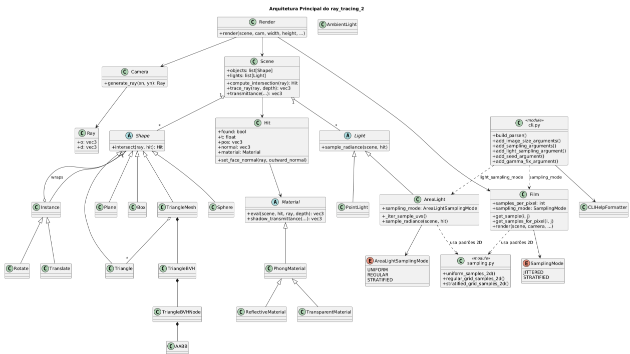
Figura 13. Diagrama de classes da arquitetura principal de ray_tracing_2 .
