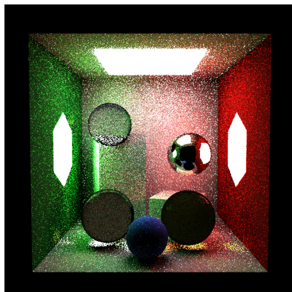
Figura 24. Cena combinada, mis em SPP=4 (depth=10, sem RR): combinação BSDF+NEE já produz imagem plausível com pouquíssimos samples ; menos ruído que bsdf_only e mais informação indireta que nee_only .
