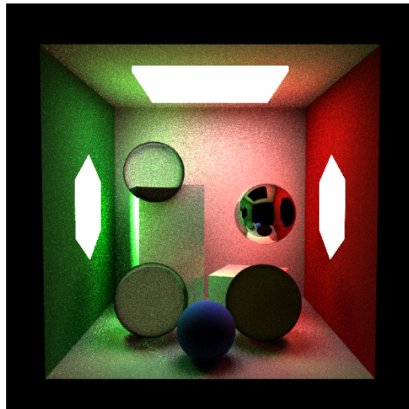
Figura 23. Cena combinada, nee_only em SPP=32 (depth=10, sem RR, 47,3 min): superfícies difusas limpas; a esfera espelhada reflete apenas geometria diretamente iluminada (sem reverberação/color bleeding).
